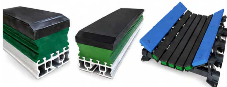
BARRAS Y CAMAS DE IMPACTO
